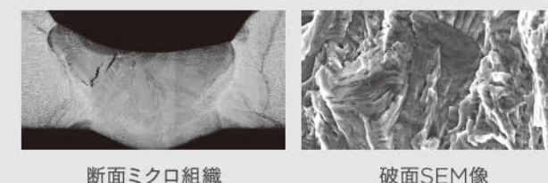
断面ミクロ組織
